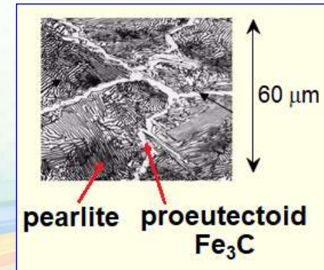
Hyperoeutectoid Steel
